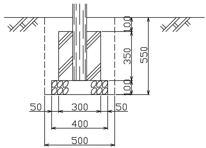
参考基礎図
