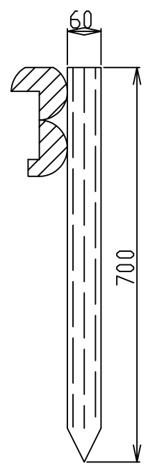
一般断面
