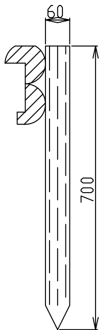
一般断面
