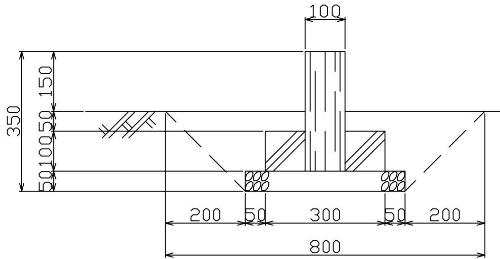
参考基礎図
