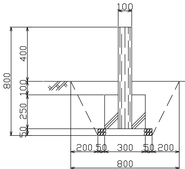
参考基礎図
