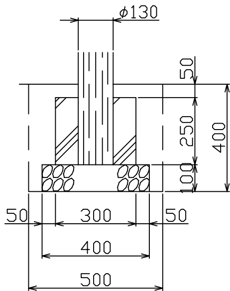
参考基礎図
