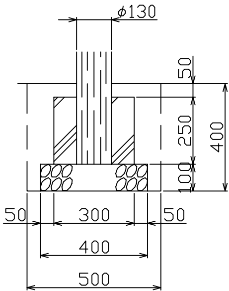
参考基礎図
