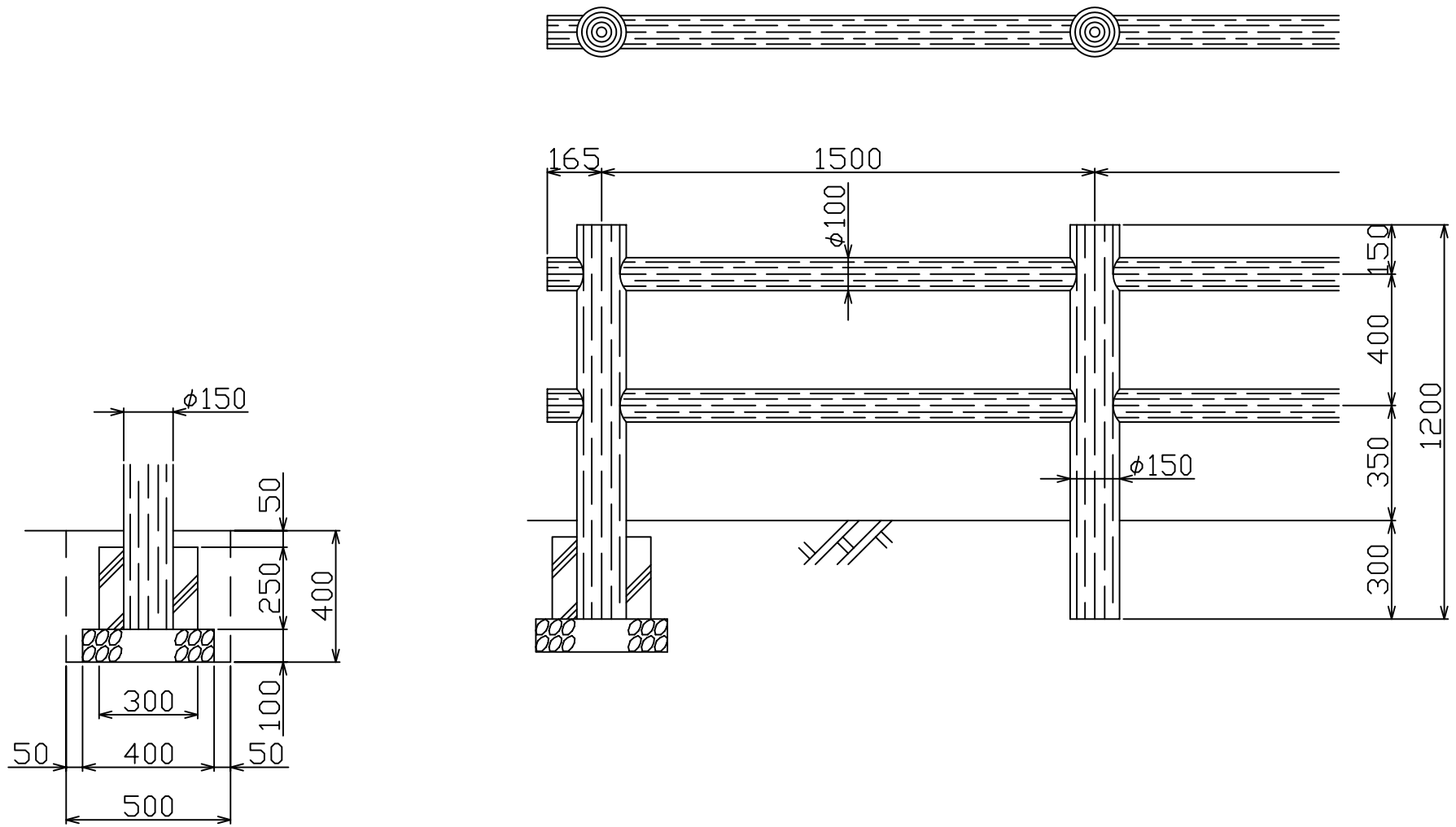
参考基礎図
