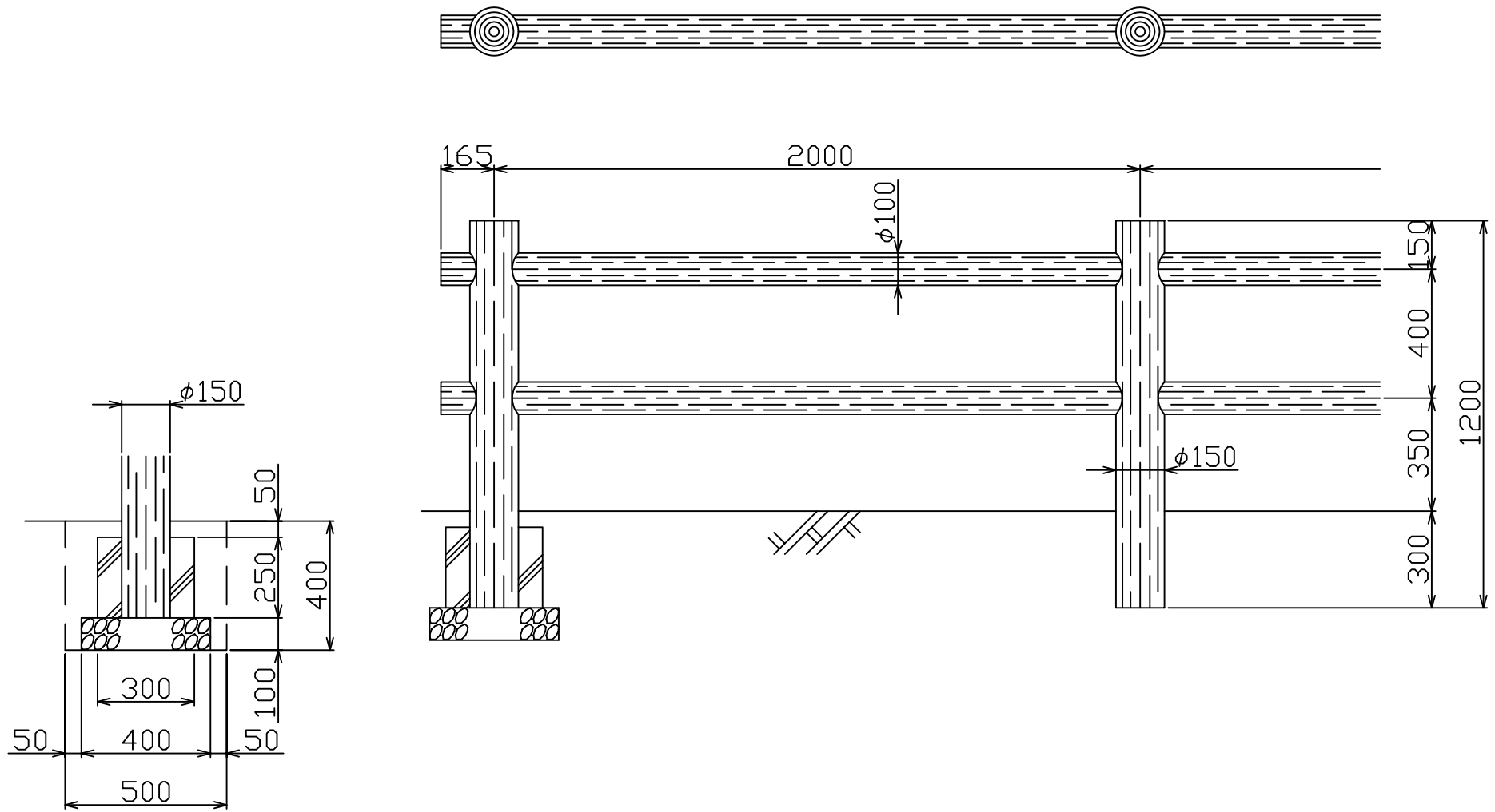
参考基礎図
