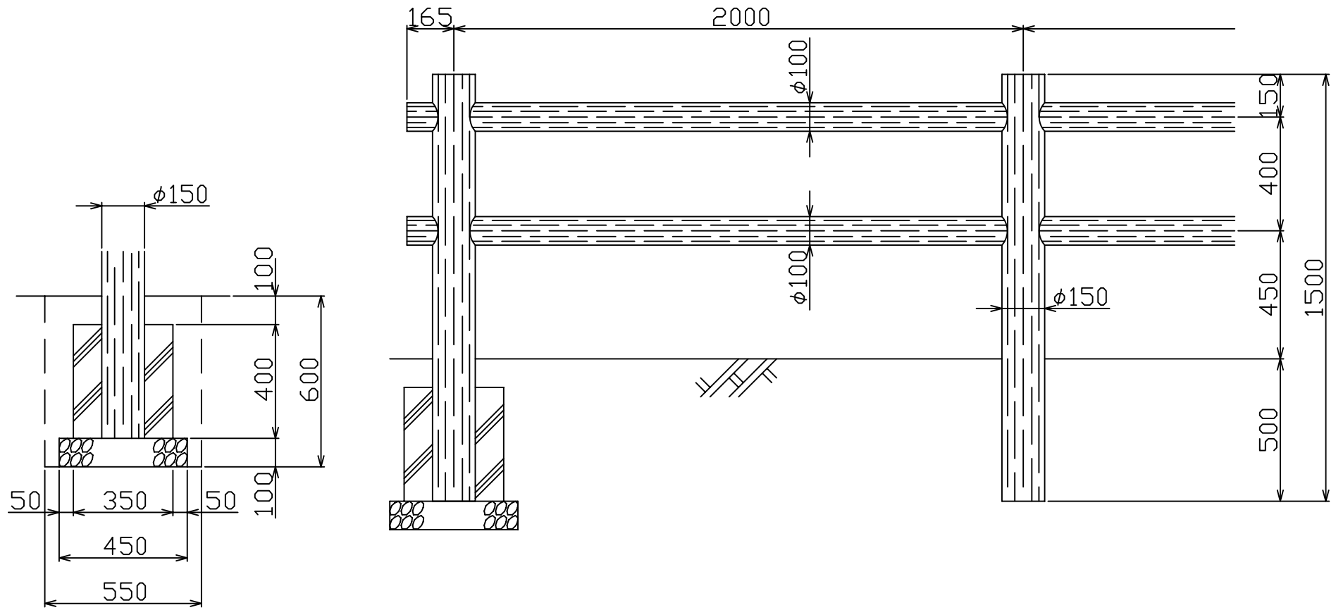
参考基礎図
