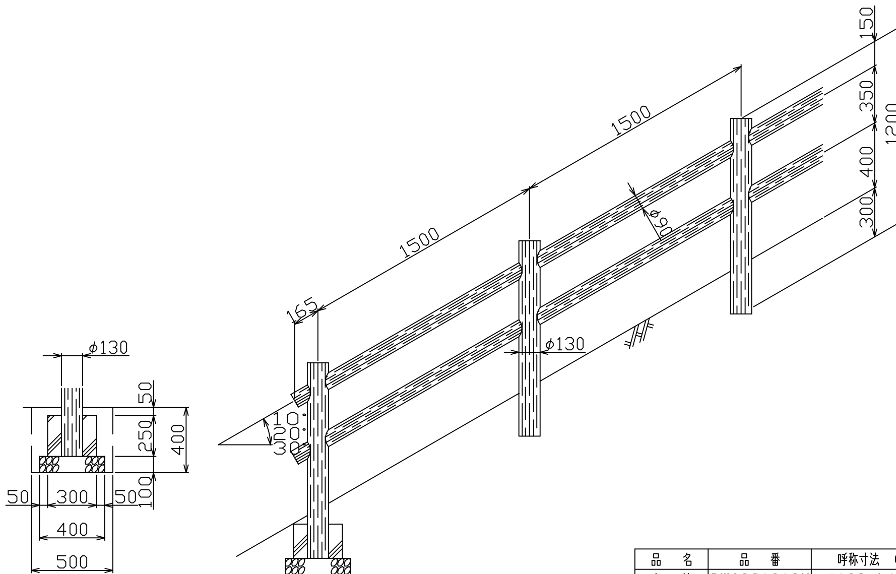
参考基礎図
