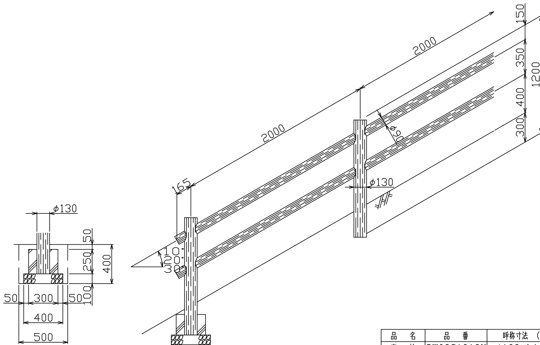
参考基礎図
