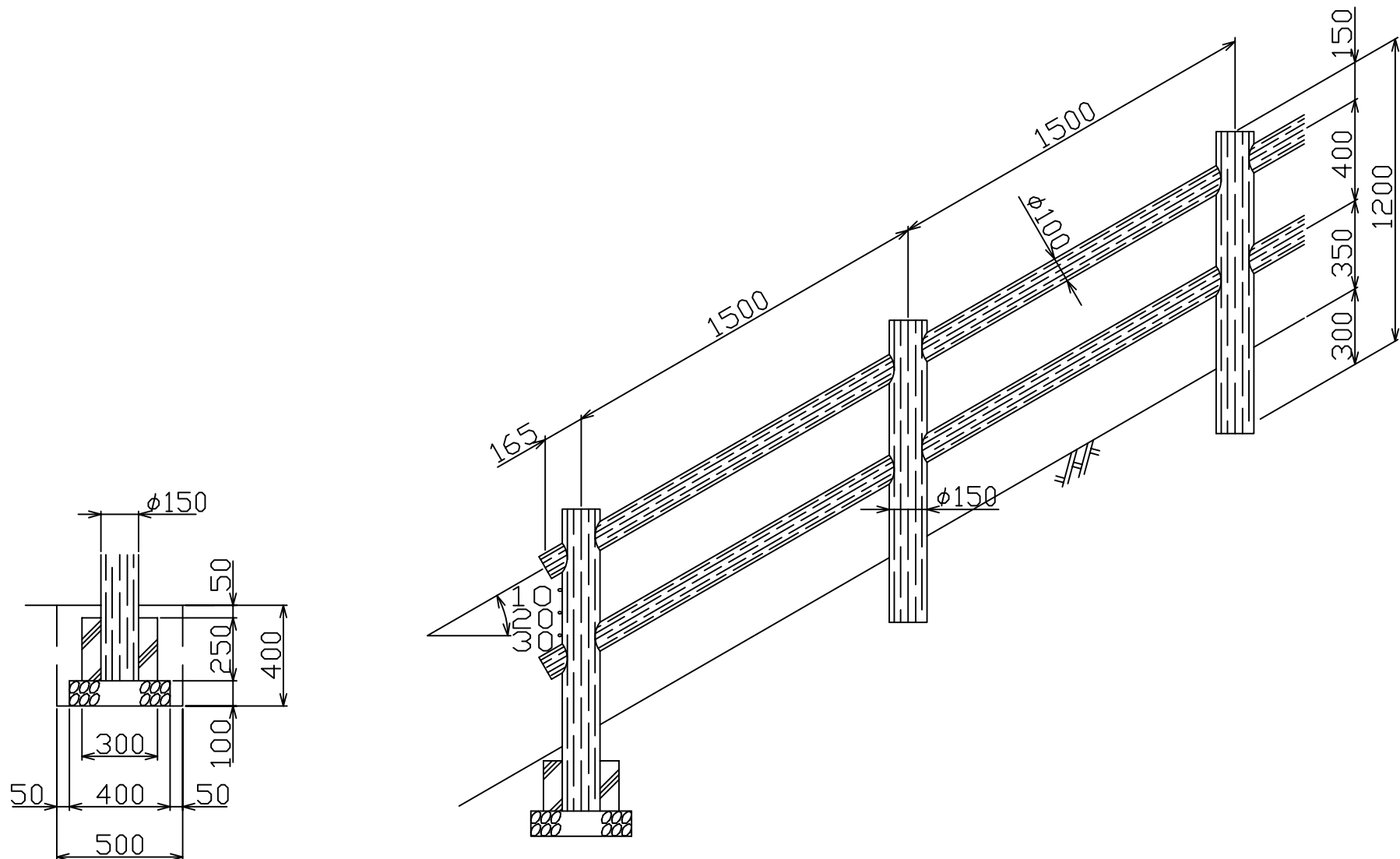
参考基礎図
