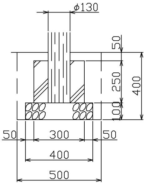
参考基礎図
