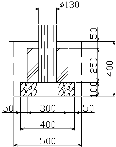
参考基礎図
