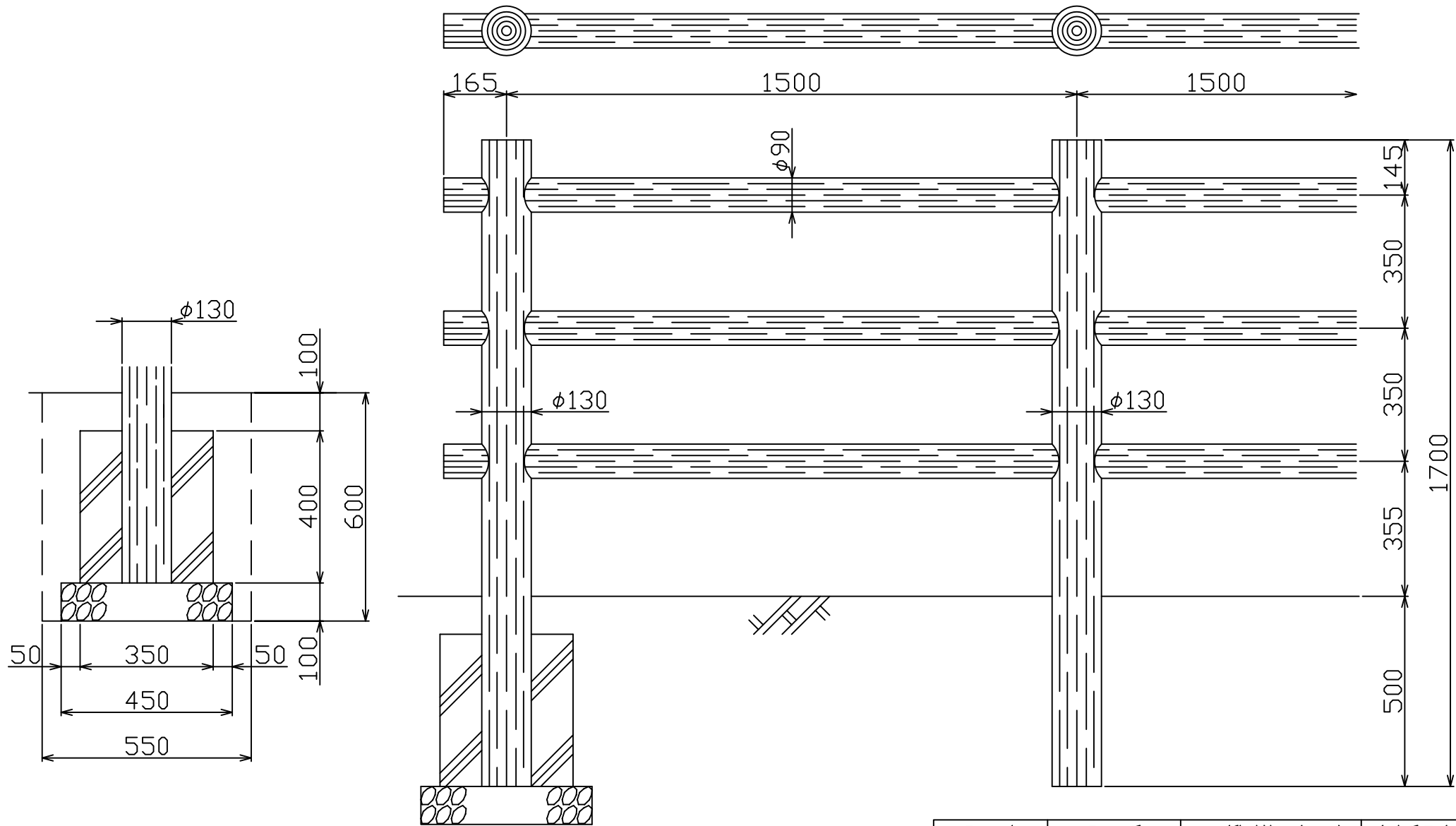
参考基礎図
