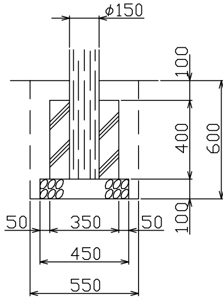
参考基礎図
