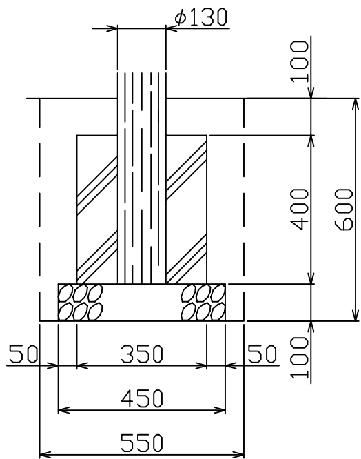
参考基礎図
